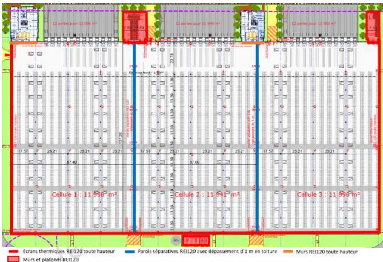
Plan 4 : Murs coupe-feu de l'entrepôt
